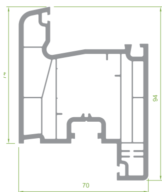
PRP.7400 Door Sash Profile
